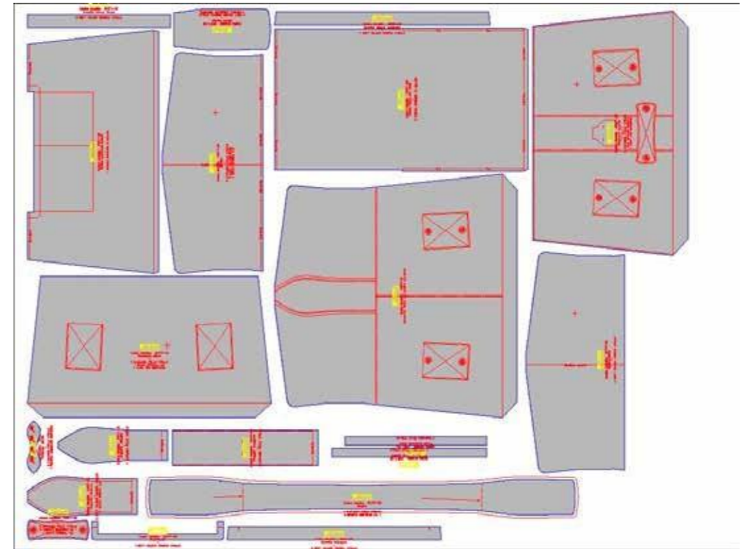
Un ejemplo de distribución automática optimizada (Nesting)
